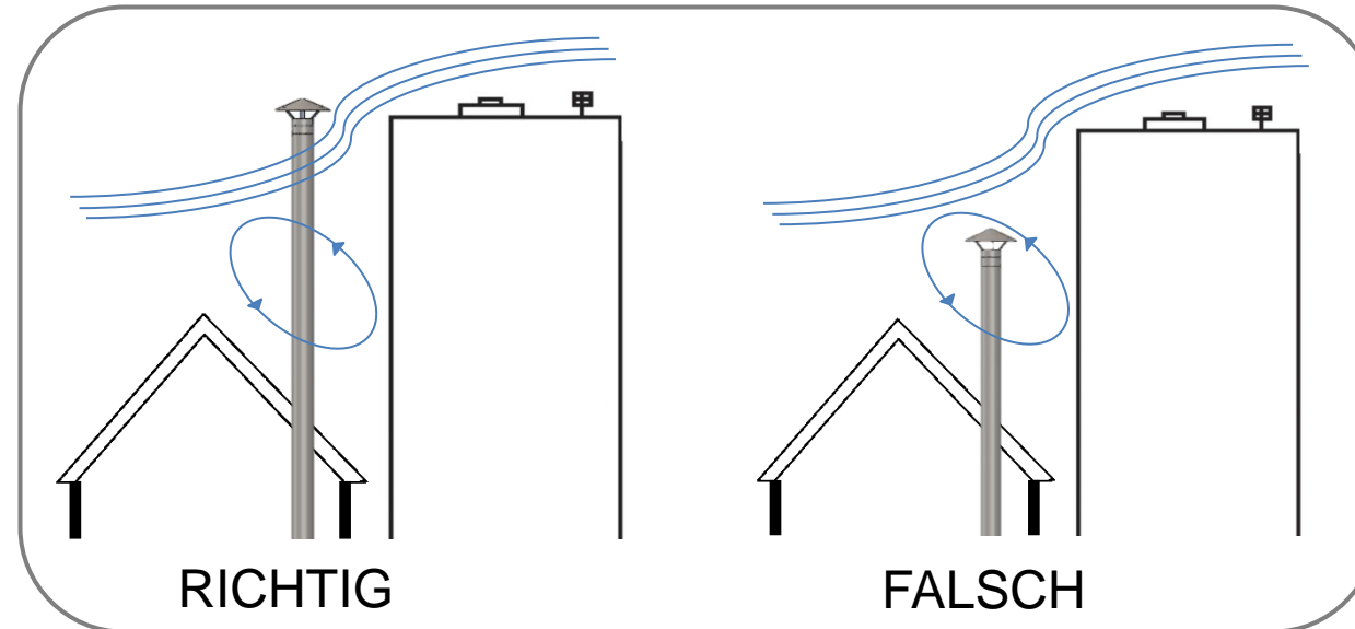
2 a Fall.- Schornstein endet überhalb der Firstpfette, jedoch unterhalb eines umliegenden Gebäudes.
