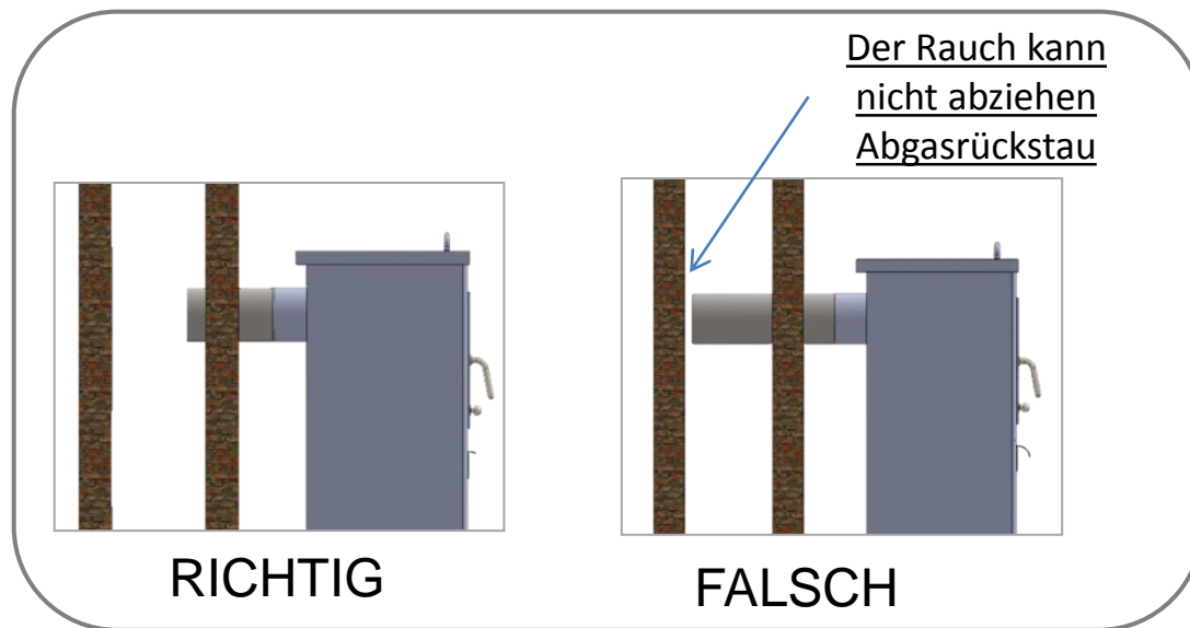
4 o Fall.- Fehlerhafte Instalation des Kaminofens- Rauchrohres.
